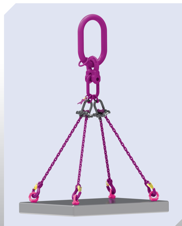
4-Strand mit Minilifter und IAK-RG 1-13 passend bis Kranhaken-Nr. 8 (DIN 15401)
