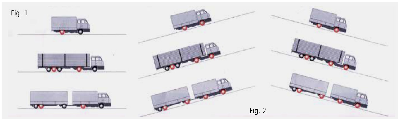
Fig. 1: Bei LKW's muss immer die angetriebene Achse bekettet werden. Bei Zugmaschinen bzw. Anhängern soll außerdem die vorletzte Achse bekettet werden. Bei Berg-/Talfahrten sollen zusätzlich die Achsen laut Fig. 2 bekettet werden.
