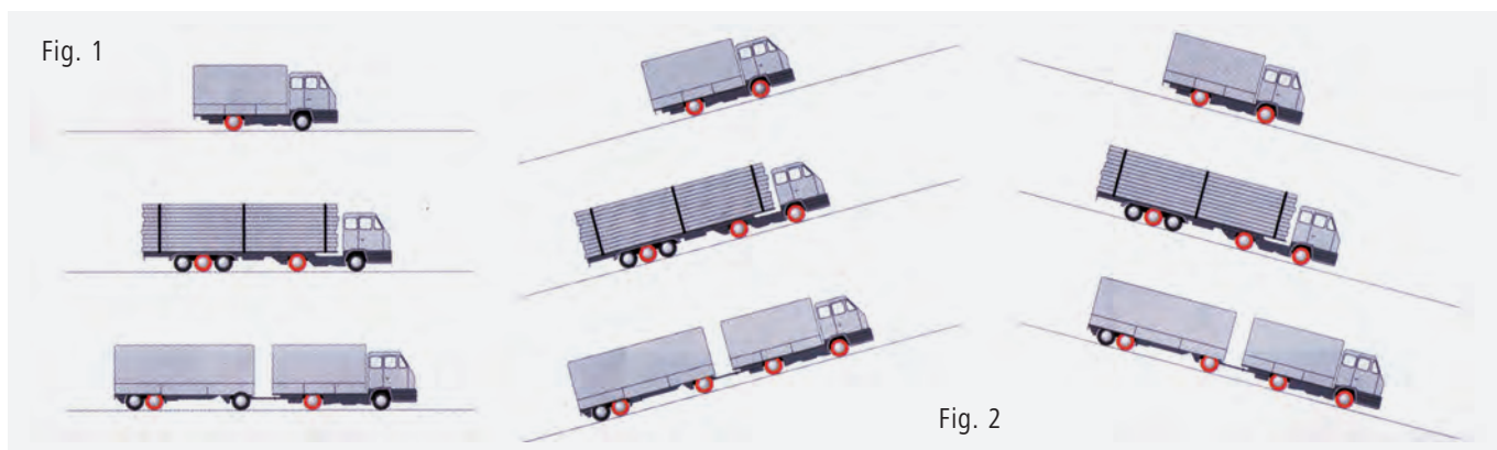
Figure 1: Sur un camion, les roues de l'essieu moteur devront toujours être équipées de chaînes. Sur les véhicules tracteurs ou les semi-remorques, les roues de l'avant-dernier essieu devront aussi être équipées. En cas de conduite en pente (montées/descentes), équiper en outre les essieux comme représenté en fig. 2 .
